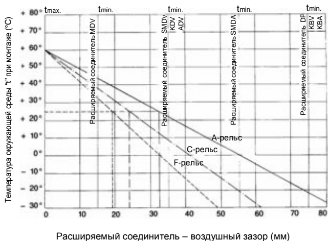
Диаграмма по установке воздушных зазоров расширяемого соединителя
